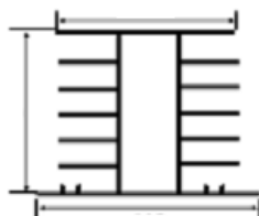
HSDS-TRI-SSR60 /80 /90 E 120A – Dissipador Trifásico Dimensões : Descritas na tabela acima
