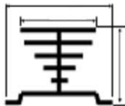
HSDS-MON-SSR15A – Dissipador Monofásico Dimensões : 80mm * 50mm * 50mm
