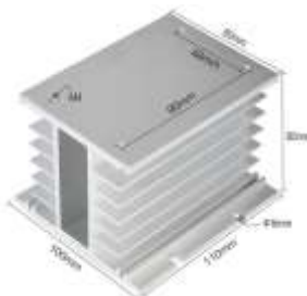
HSDS-TRI-SSR60 /80 /90 E 120A – Dissipador Trifásico Dimensões : Descritas na tabela acima
